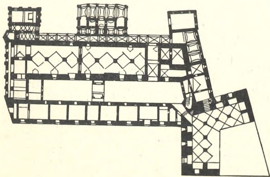
Tločrt mariborskega mestnega gradu iz leta 1933
