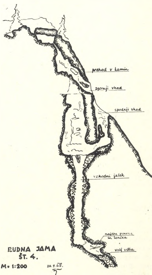
Prerez rudne jame št. 4 v območju Planic na robu Jelovice zahodno od Krope. Raziskovalca Filip Legat in inženir Janez Smitsek, ki je jamo zrisal
