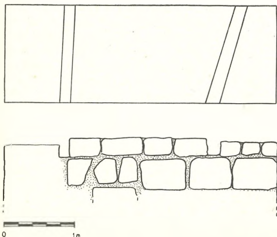
Tloris in stranski pogled na temelj pri 7,50 m
