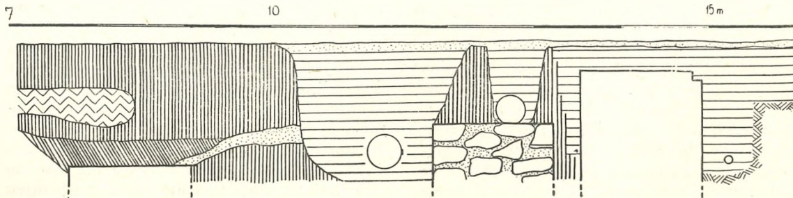
Prerez zemeljskih plasti v jarku vzhodno od gotskega stolpa med metroma 7 in 16
