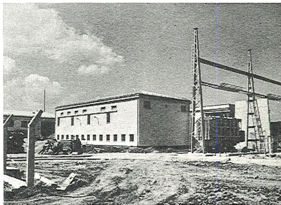
RTP Logatec. 20 KV stikališče med gradnjo
